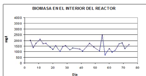
Figura 10 Biomasa en el tratamiento anaerobio en continuo
