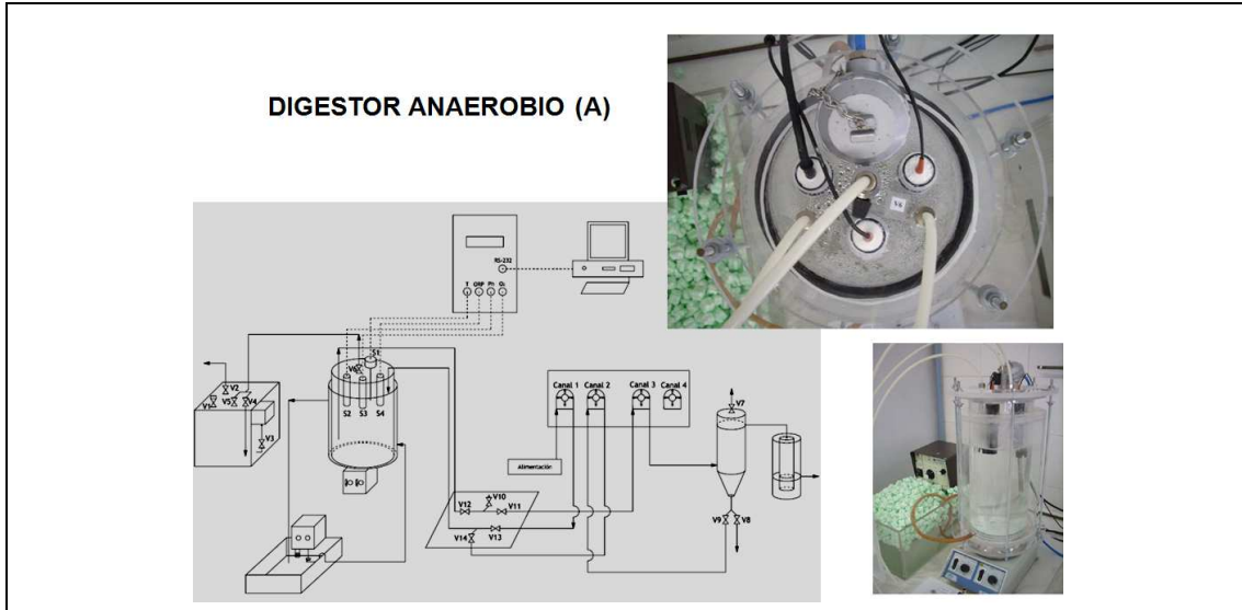
Figura 7 Diseño y construcción de las instalaciones
