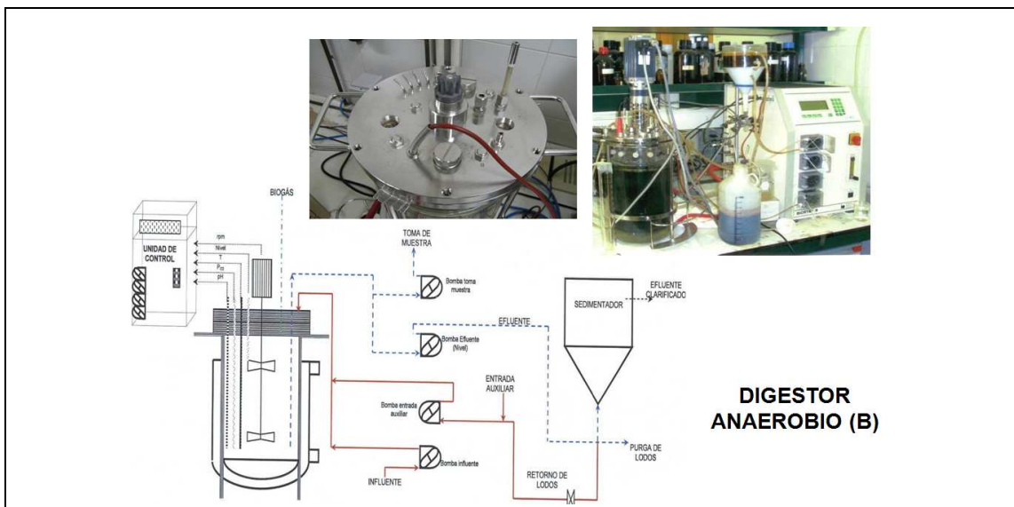
Figura 8 Diseño y construcción de las instalaciones
